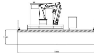
VISTA FRONTALE
